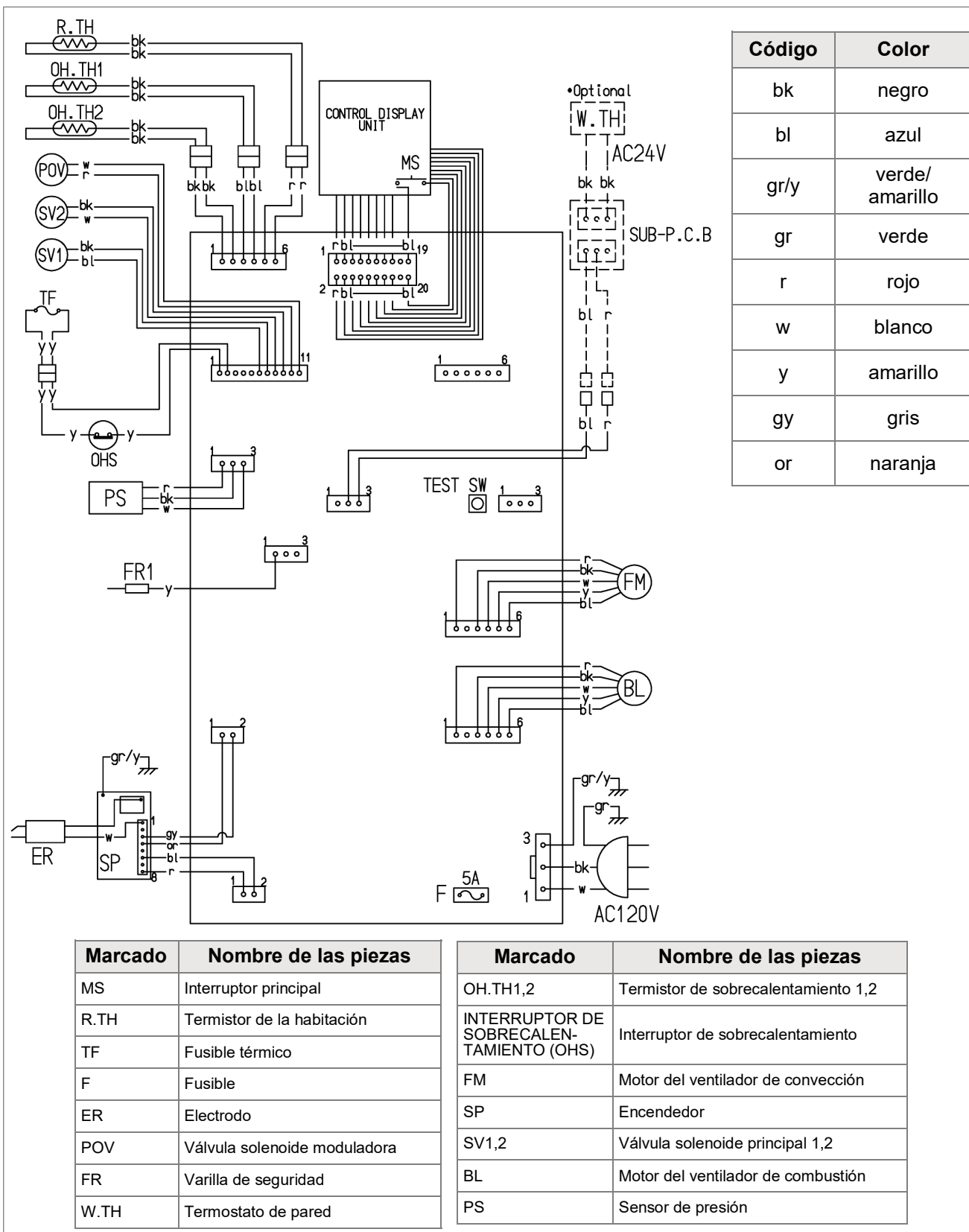
Figura 59. Diagrama de conexionado
