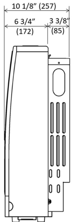
Figura 4. Vista lateral
