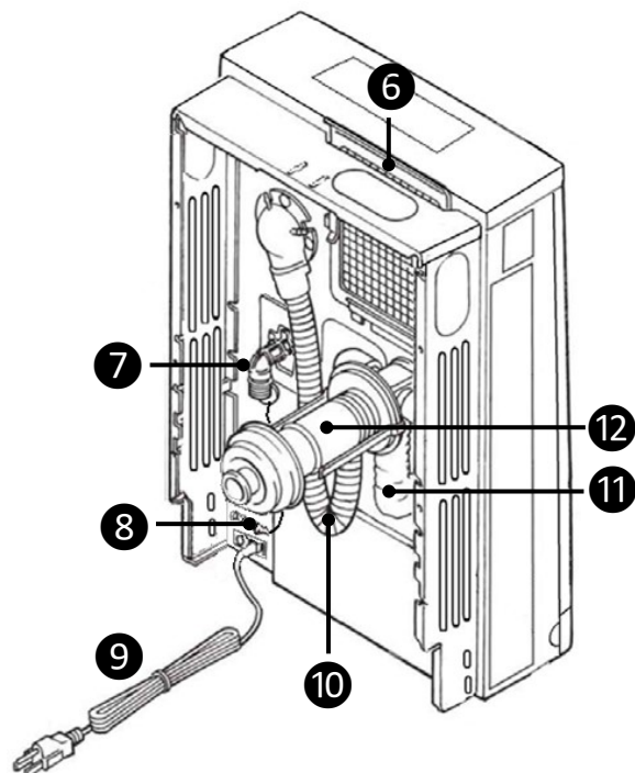
Figura 2. Vista posterior
