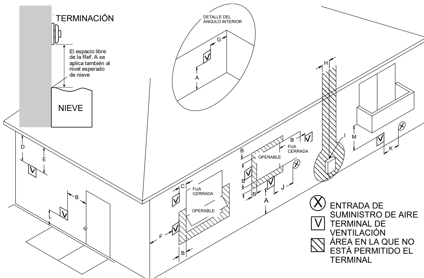
Figura 5. Espacios libres del terminal del conducto de humos
