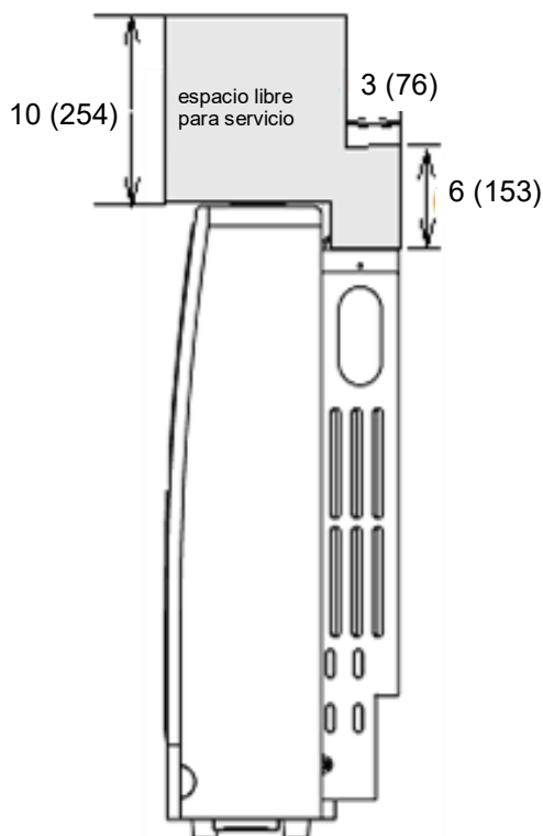
Figura 7. Espacios libres recomendados para tareas de servicio
