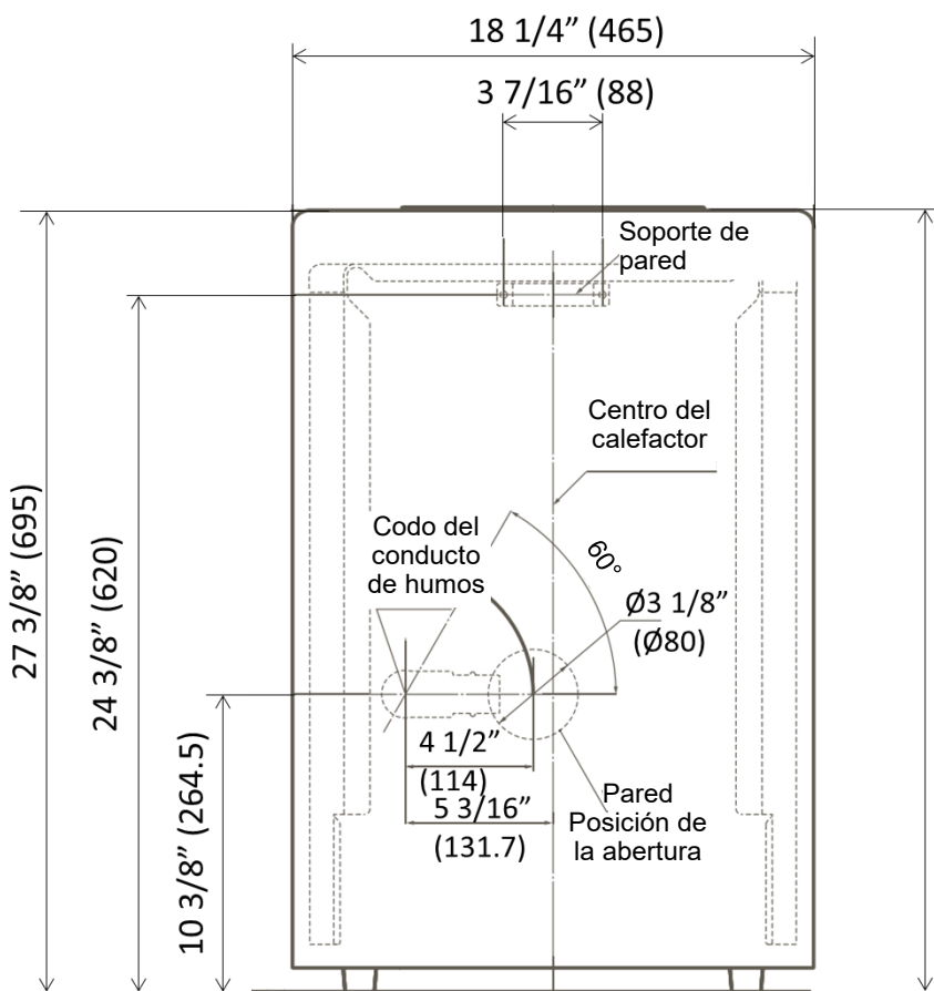
Figura 3. Vista frontal
